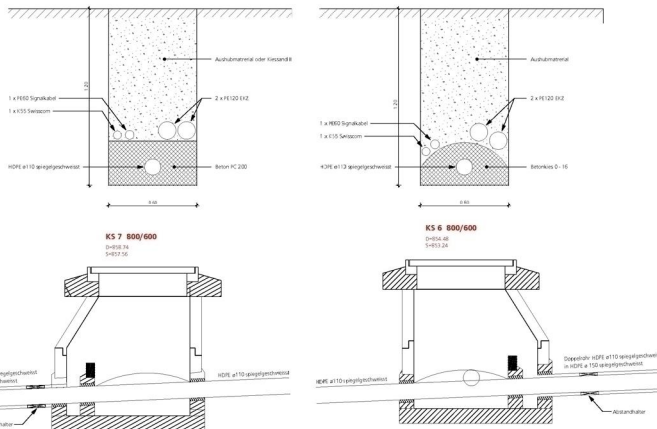
Grabenprofile und Schachtdetails
