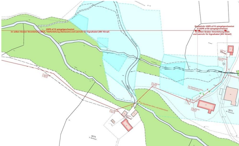
Situation Bauprojekt
