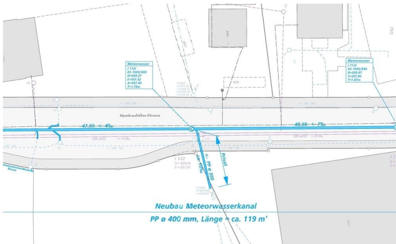
Ausschnitt Ausführungsplan
