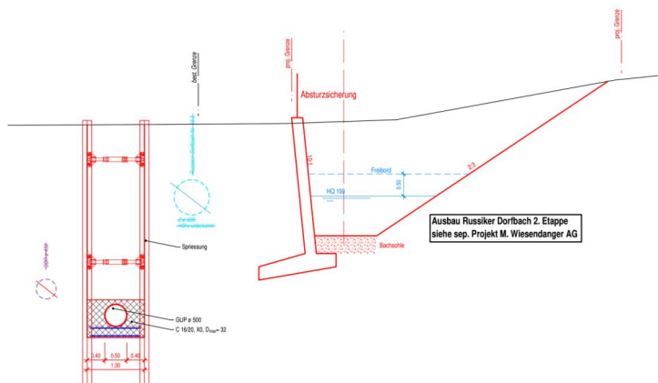
Grabenprofil mit Verlegung Dorfbach Russikon 2. Etappe
