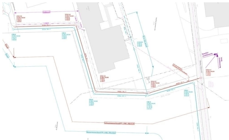
Situation Ausführungsprojekt
