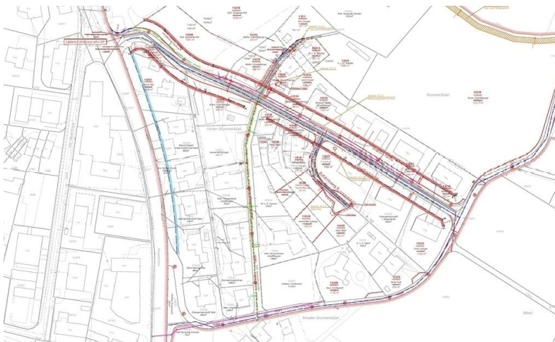
Ausschnitt Werkleitungen/Baulinien
