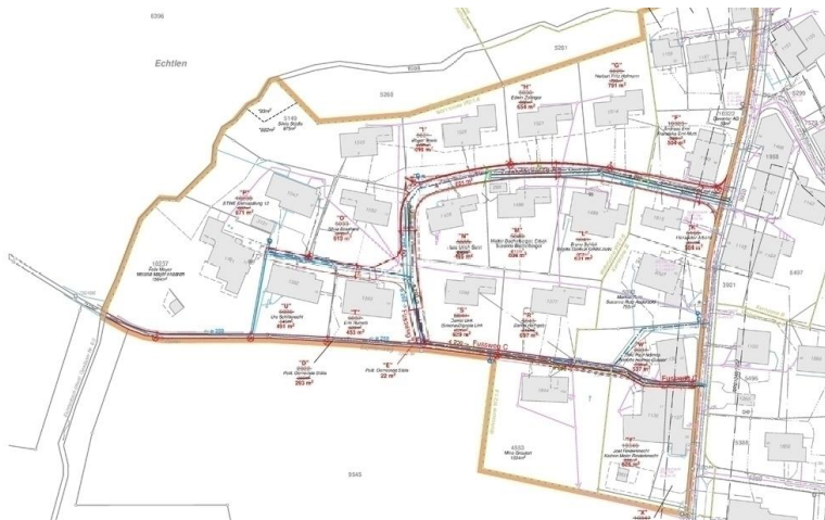
Situation Werkleitungen Quartierplanentwurf
