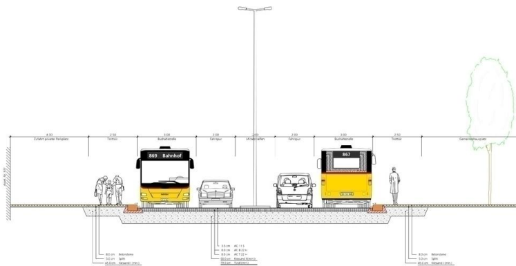
Querschnitt Madetswilerstrasse mit neuer Bushaltestelle
