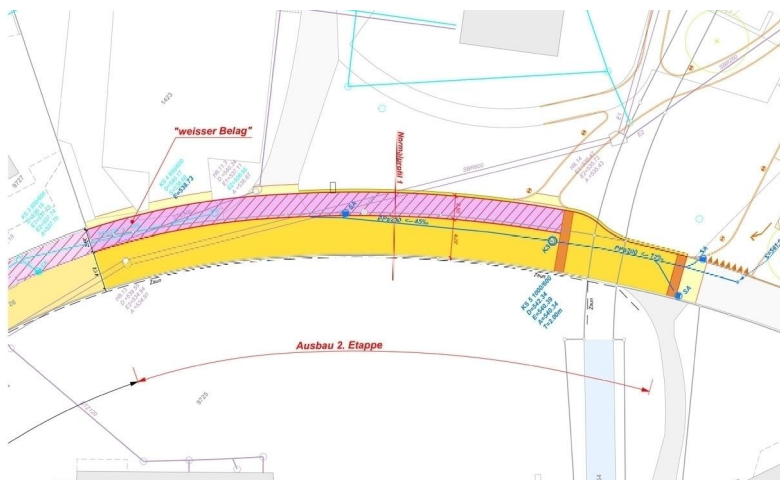
Situation Ausführungsplan
