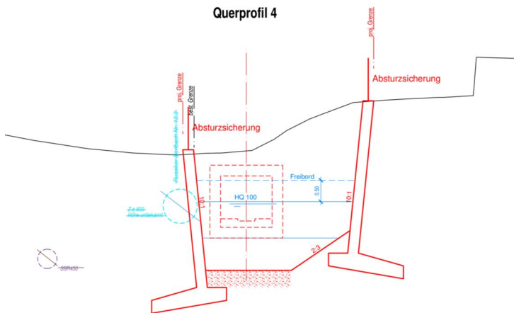
Querschnitt Bachausbau
