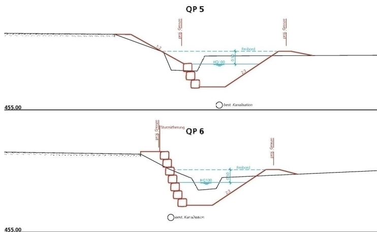
Auszug aus dem Querprofilplan
