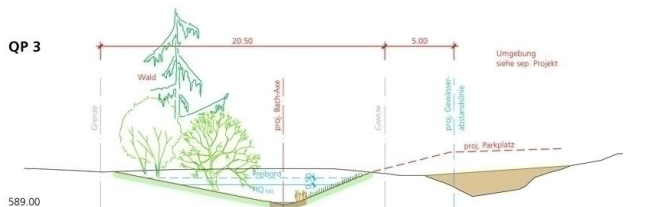
Querprofile
